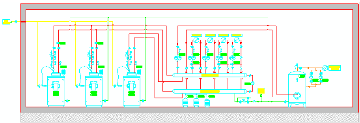
Figura 4.7 - Particolare dello schema di impianto
