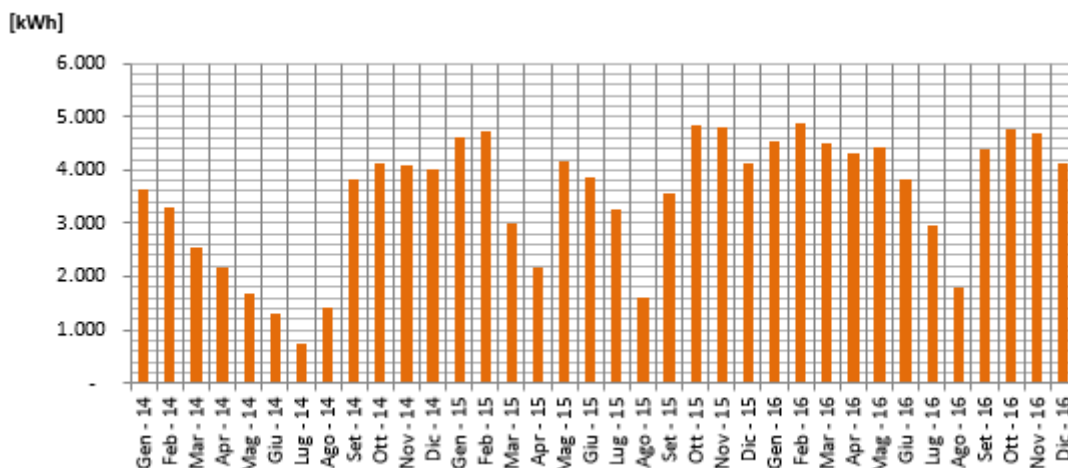
Figura 5.1 – Confronto tra i profili elettrici reali relativi a ciascun POD per il triennio di riferimento
